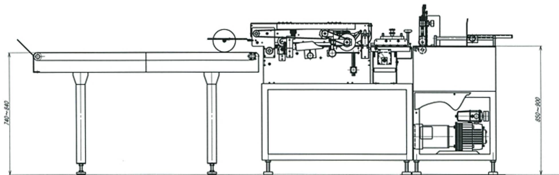
高速自動封緘機機器構成図
